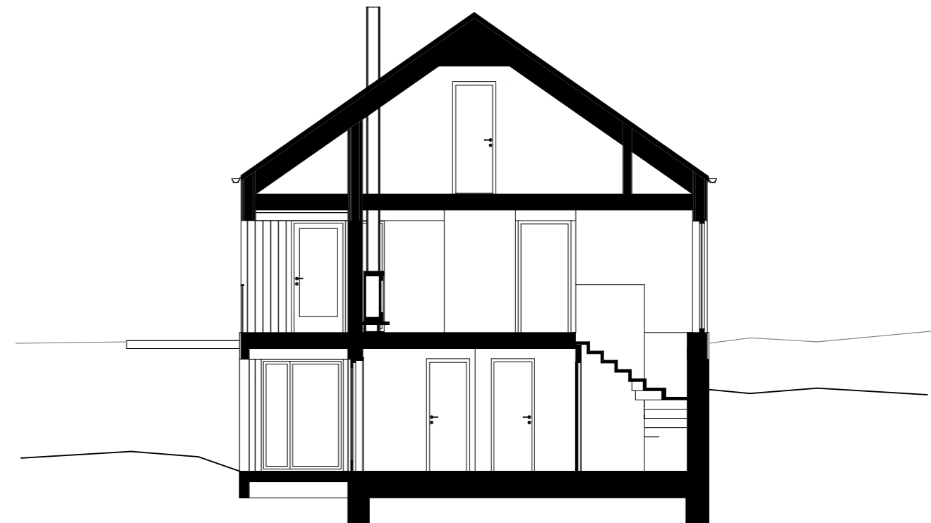
TVERRSNITT AA
